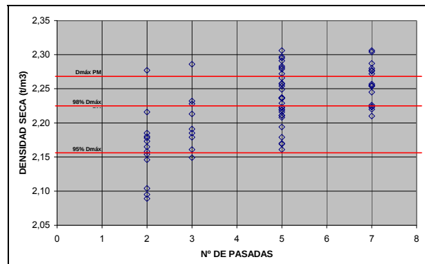
Figura 1.- Densidad seca en función del número de pasadas (1ª campaña)
