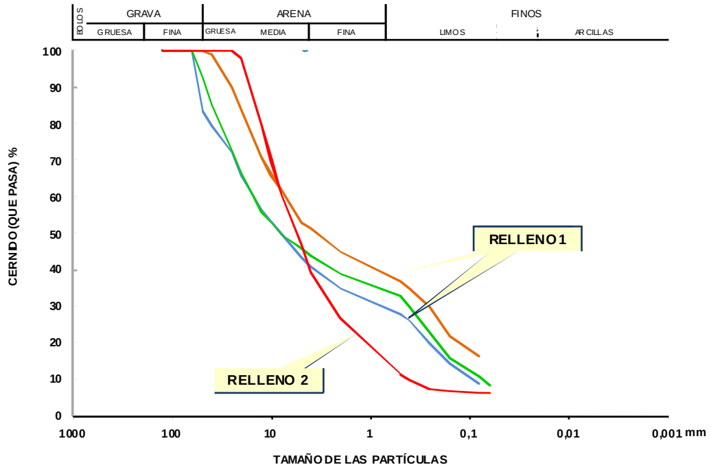
Figura 1.- Curvas granulométricas del material ensayado
