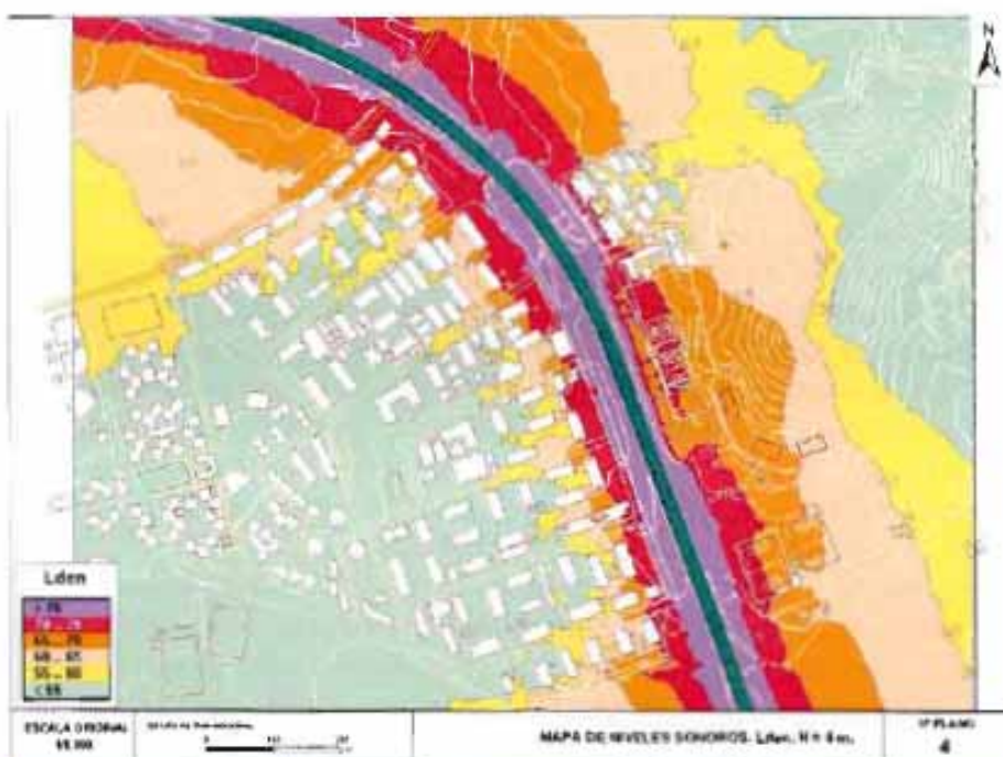
Gráfico 3. Mapa de niveles sonoros L_{den} , Fase B
