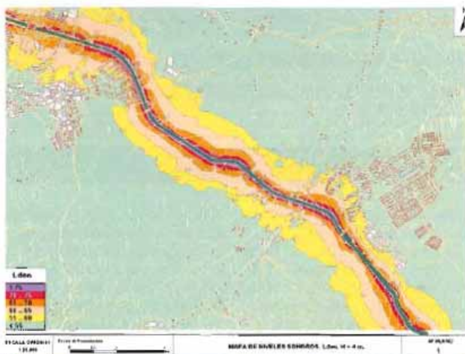
Gráfico 2. Mapa de niveles sonoros L_{den} , Fase A
