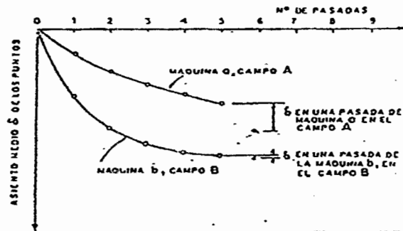
ASIENTO MEDIO DE UNA TONGADA EN FUNCION DEL N° DE PASADAS DE DOS MAQUINAS DE COMPACTACION.
