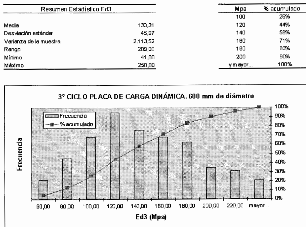
Figura.13. Resumen estadístico de Ed3 con placa de carga dinámica. Suelo estabilizado con cemento
